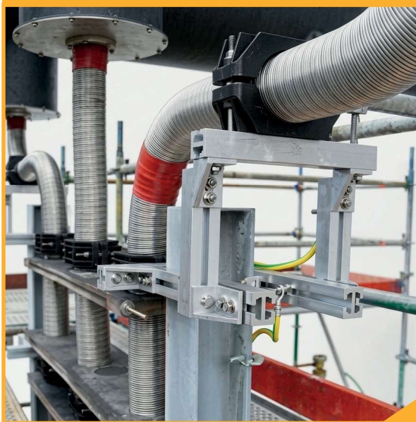
Conexión SIS a IPB
