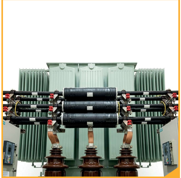
Conexión de aparamenta con aislamiento de gas
