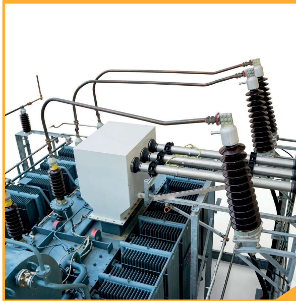
Conexión SIS al transformador con caja de protección
